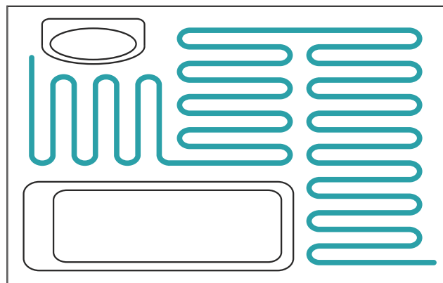
Ilustračný obrázok rozloženia elektrického kúrenia.
