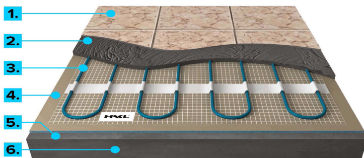
Ilustračný obrázok zloženia podlahy
